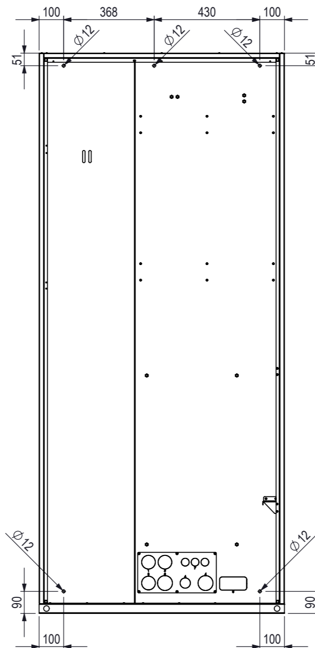
DETTAGLIO FISSAGGIO A PARETE
