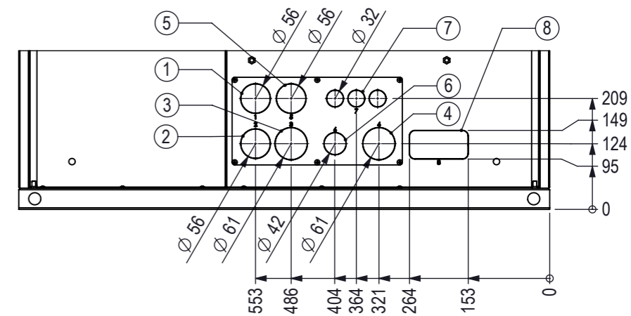
DETTAGLIO INGRESSO TUBAZIONI DAL POSTERIORE
