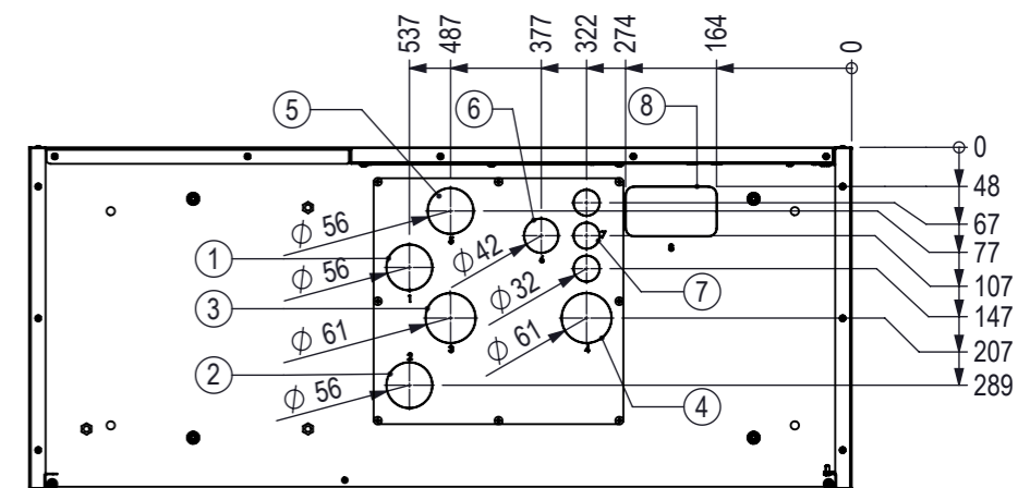
DETTAGLIO INGRESSO TUBAZIONI DAL FONDO
